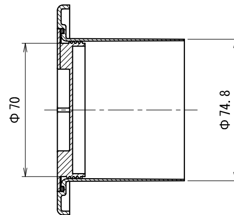
断面 A-A
